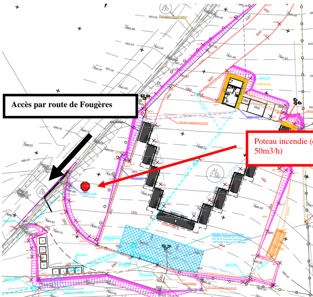
Extrait du plan de masse (Récolement entreprise Colas – 2011)
